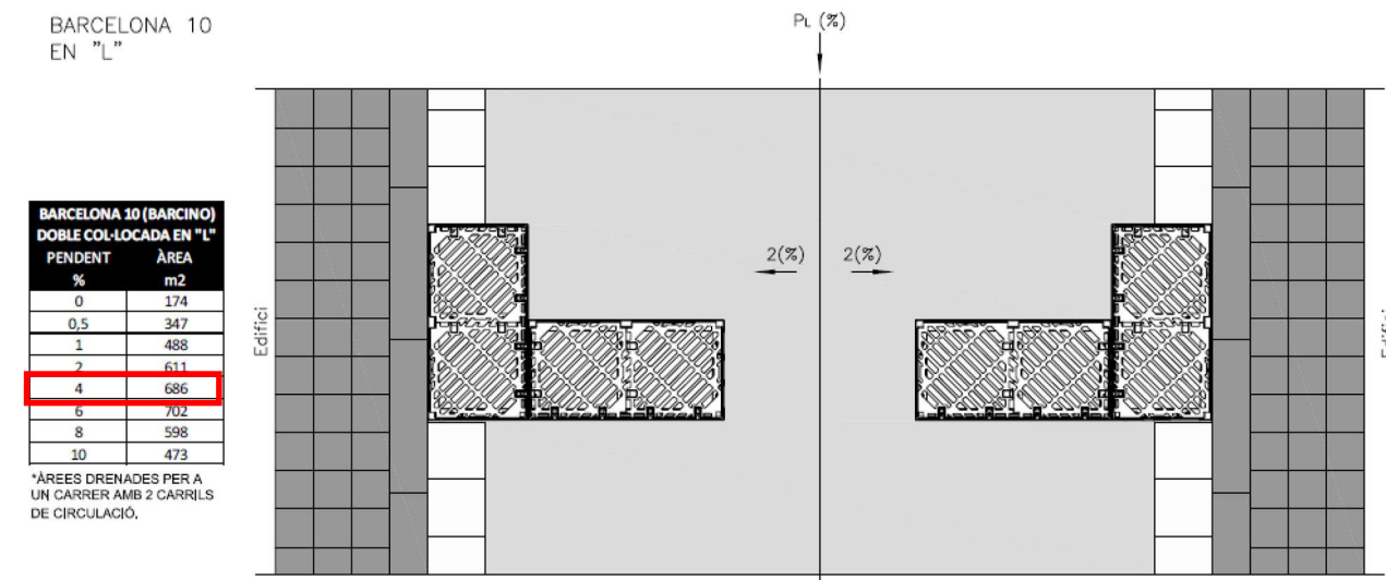
Figura 1. Taules de capacitat d'embornals projectats a calçada.
