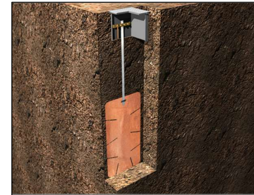
Imatge 2. Representació de presa a terra a instal·lar
