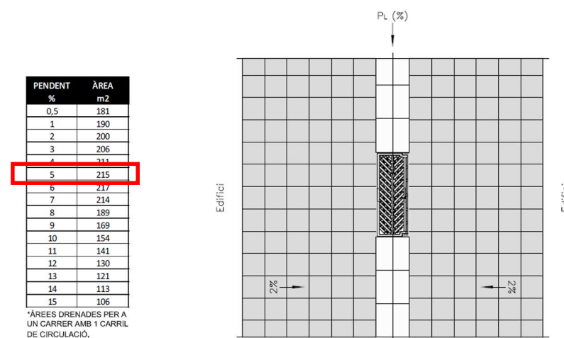
Figura 2. Taules de capacitat d'embornals projectats a carrers peatonals.
