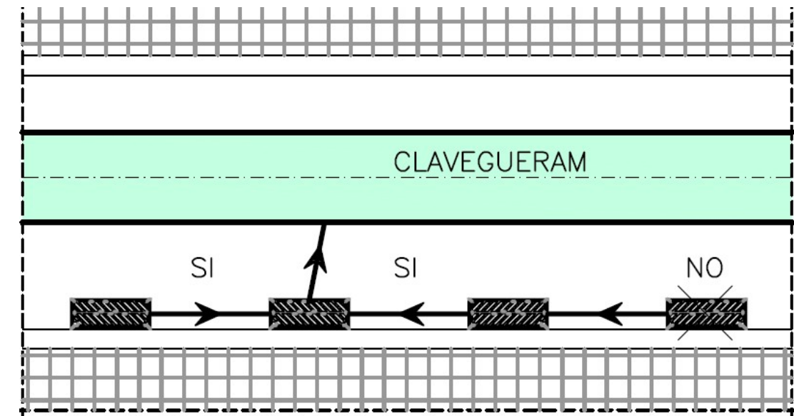
Figura 1. Esquema de disposició d'embornals i connexions.
