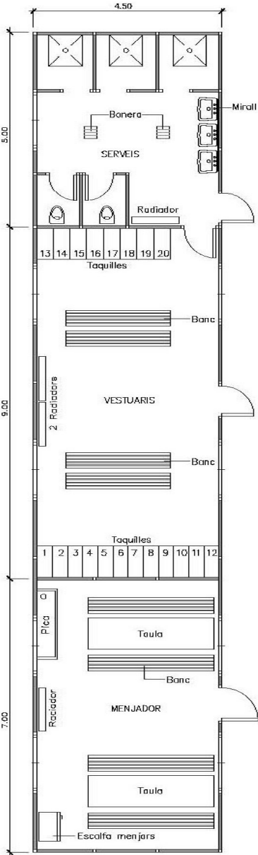
Planta barracons tipus
