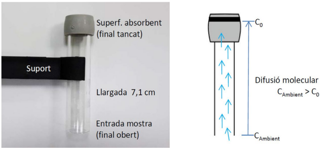
Figura 15. Principi de funcionament dels tub passius de difusió de \text{NO}_2 de tipus Palmes, on C_{\text{Ambient}} és la concentració de la mostra ambiental i C_0 és la concentració a la superfície de l'absorbent.
